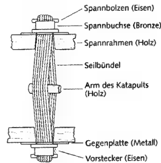
Torsionsfeder eines Katapultes (schematisch).
